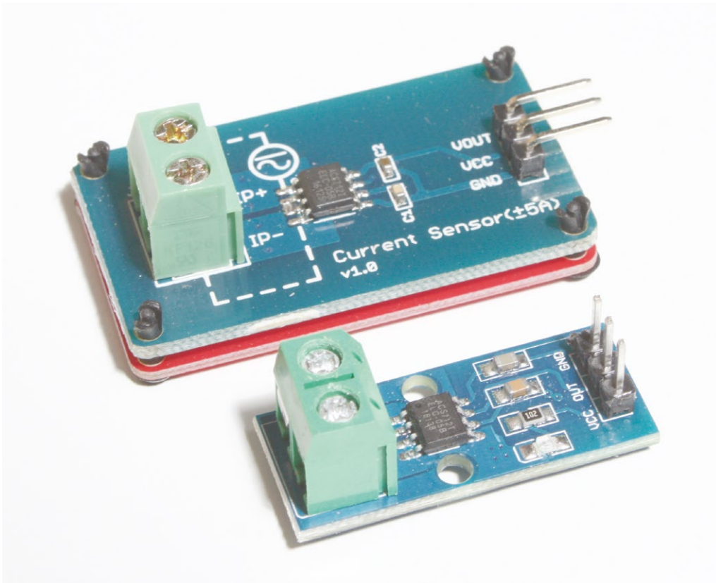
Fig. 7 : Ces deux modules sont à base d'ACS712. Le plus gros avec une plaque d'isolation (en haut) est celui qui a donné les meilleurs résultats lors de nos expérimentations (voir la mise en pratique plus loin dans cet article). On le trouve pour un peu moins de 5 euros chez Deal Extreme ( www.dx.com ).
