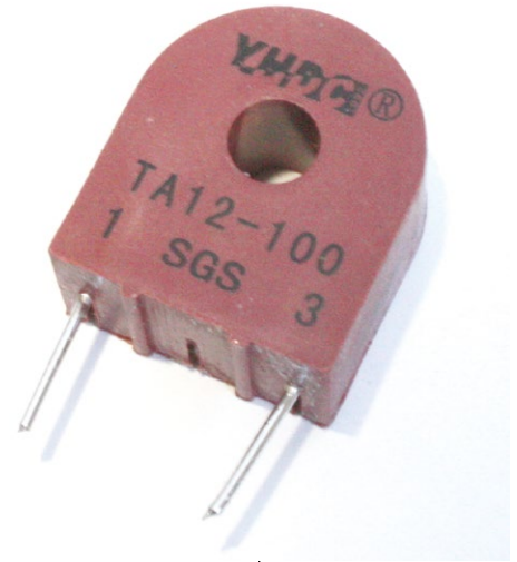
Fig. 5 : Un capteur de courant TA12-100. On le trouve souvent monté sur une breakout board, avec une simple résistance de charge, pour deux fois le prix du composant seul comme ici.
