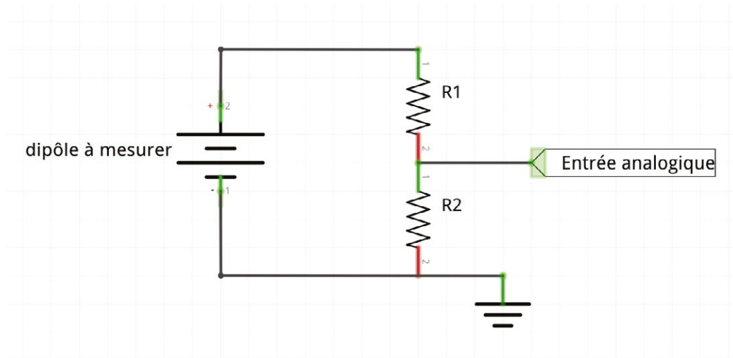
Fig.1 : Schéma d'un pont diviseur. Le dipôle peut être indifféremment un générateur (batterie, transformateur, etc.), ou bien un composant dans un circuit alimenté.
