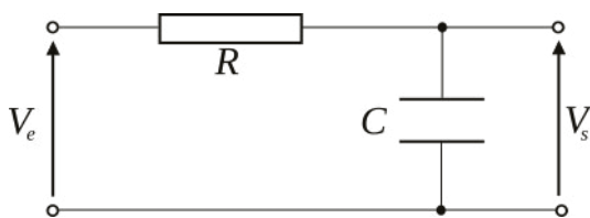
Fig. 3 : Schéma d'un filtre passe-bas.
