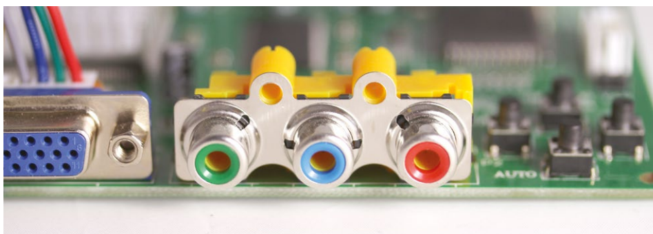
Ce connecteur composé de trois prises RCA, sur le GBS-8200, n'est pas destiné à recevoir un signal RGB, mais YUV (YPbPr) et ce malgré le fait que les connecteurs soient effectivement rouge, vert et bleu. L'entrée RGB, elle, se présente sous forme de broche, ailleurs sur le circuit.
