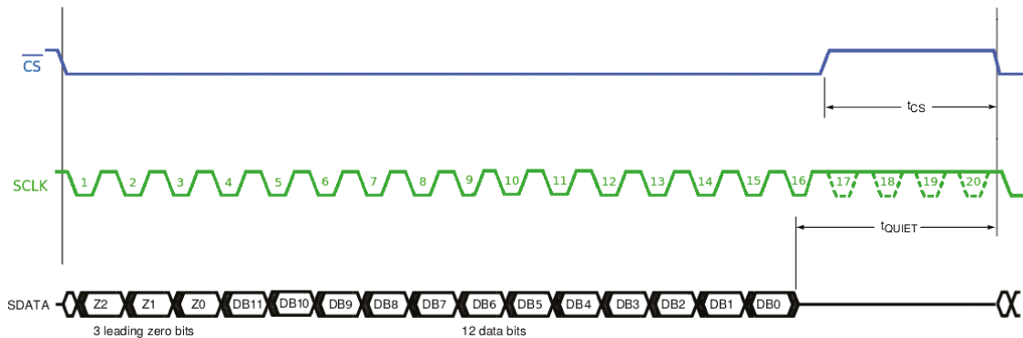
Le chronogramme débarrassé du superflu.
