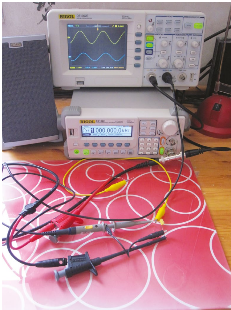
Fig. 1 : Les appareils en situation avec un filtre RC câblé « en l'air ».
